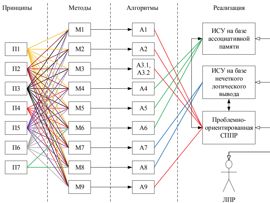
Рис. 1. Методология поддержки принятия решений при интеллектуальном управлении ТСПП
