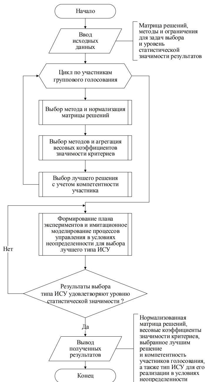
Рис. 3. Алгоритмическое обеспечение проблемно-ориентированной СППР
