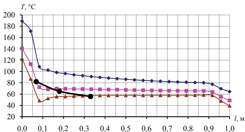
Рис. 5. Зависимость температуры стенки кристаллизатора по высоте слитка:
